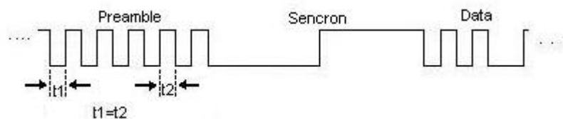
Şekil 3. Data Format
